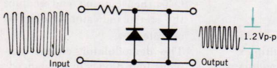
Fig. 1-1 Diode limiter
