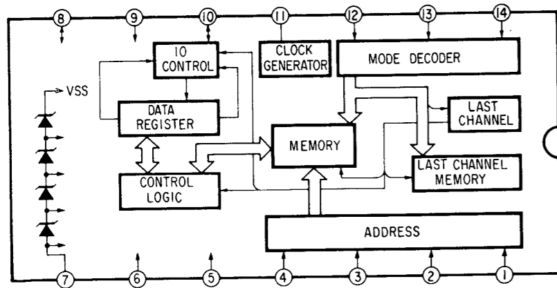
IC703 CX761A
