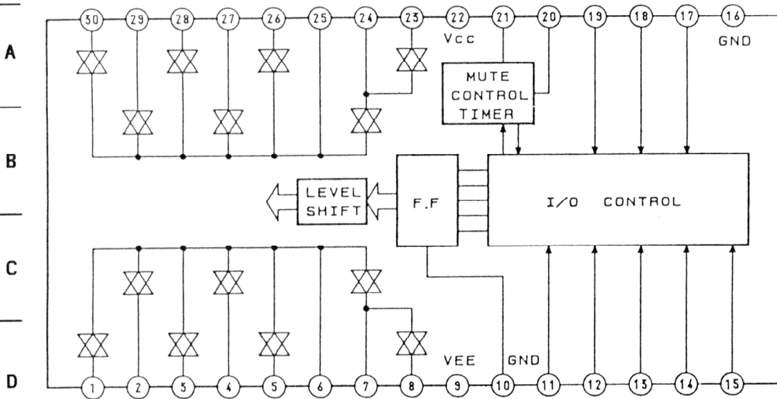
IC103 LC7818
