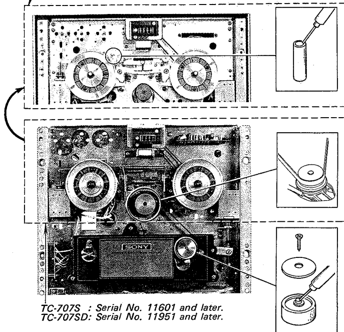
Fig. 3-2-1. Lubrication
