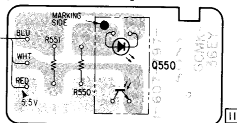
【INTERRUPT BOARD】
