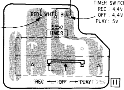
【TIMER BOARD】
