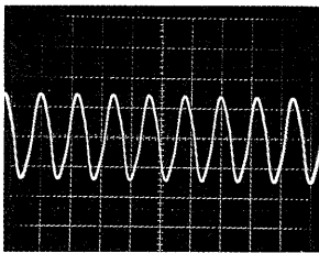
9 IC351 ④⑥pin (OSC2) 5.8Vp-p, 0.24μsec
