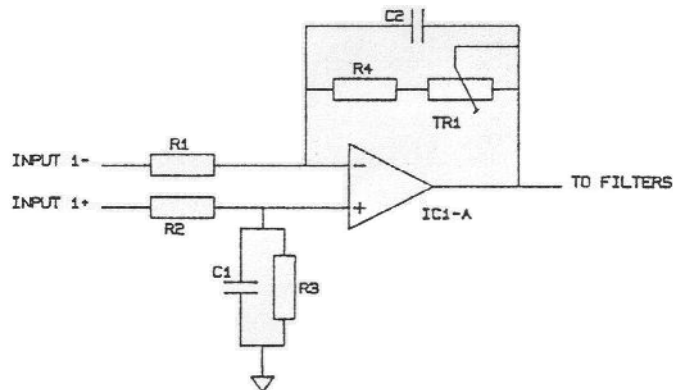
Fig 3 Input amplifier
