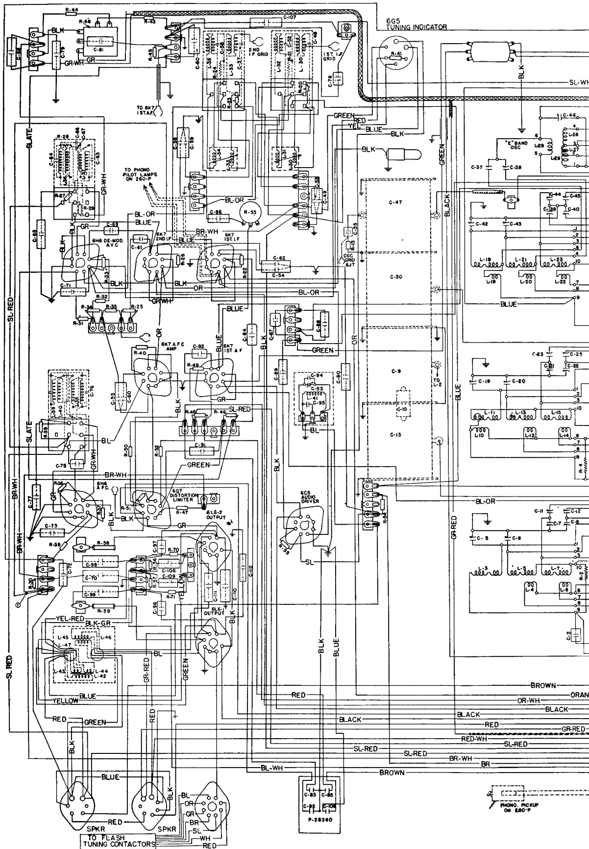
Fig. 4. Wiring Diagram.
