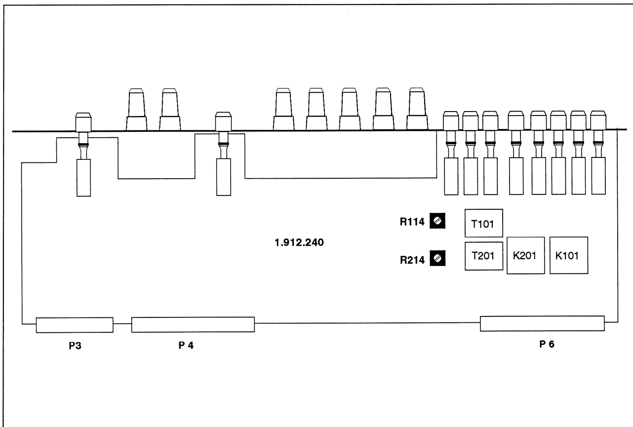
Fig. 11 Abgleichelemente der Eingangseinheiten Stereo Hochpegel Version "A".
