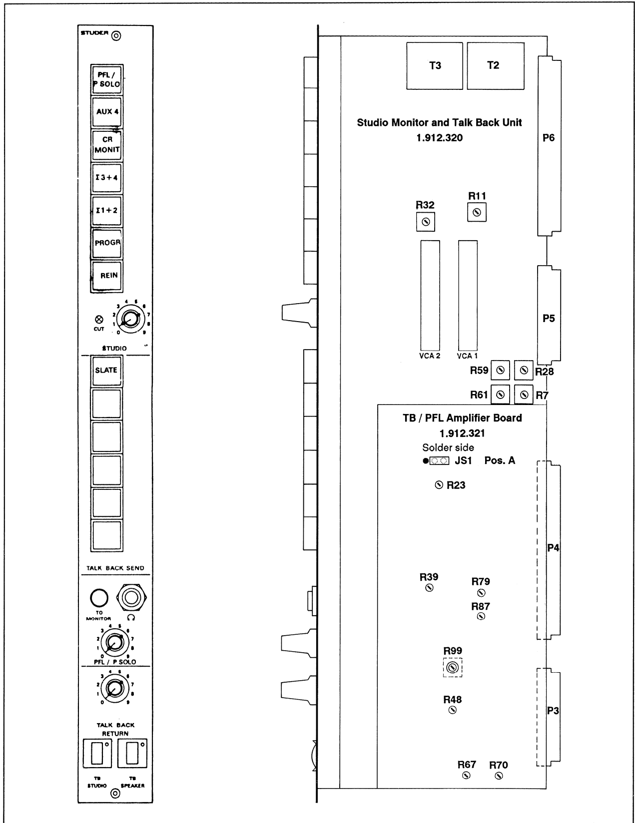
Fig. 19 Abgleichelemente der Studio Monitor und Kommando-Einheit 1.912.320.
