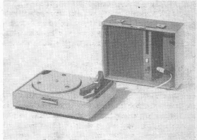
Obr. 1. Kufríkový gramofon se zesilovačem
