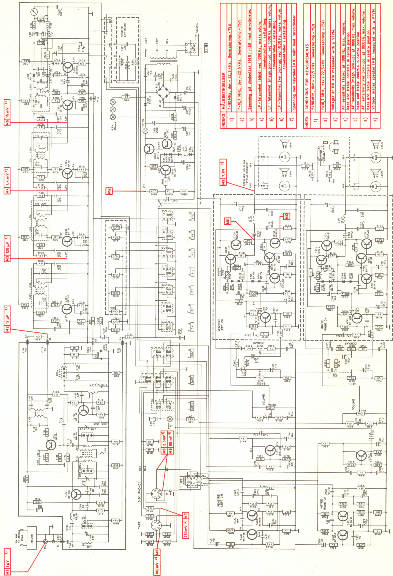
Fig. 9. Skjema for HiFi-FM Schematic HiFi-FM
