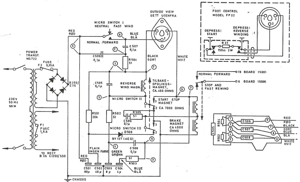
Skjema for fjernstyringsenhet modell 15 F. Under serienr. 2 510 020.
