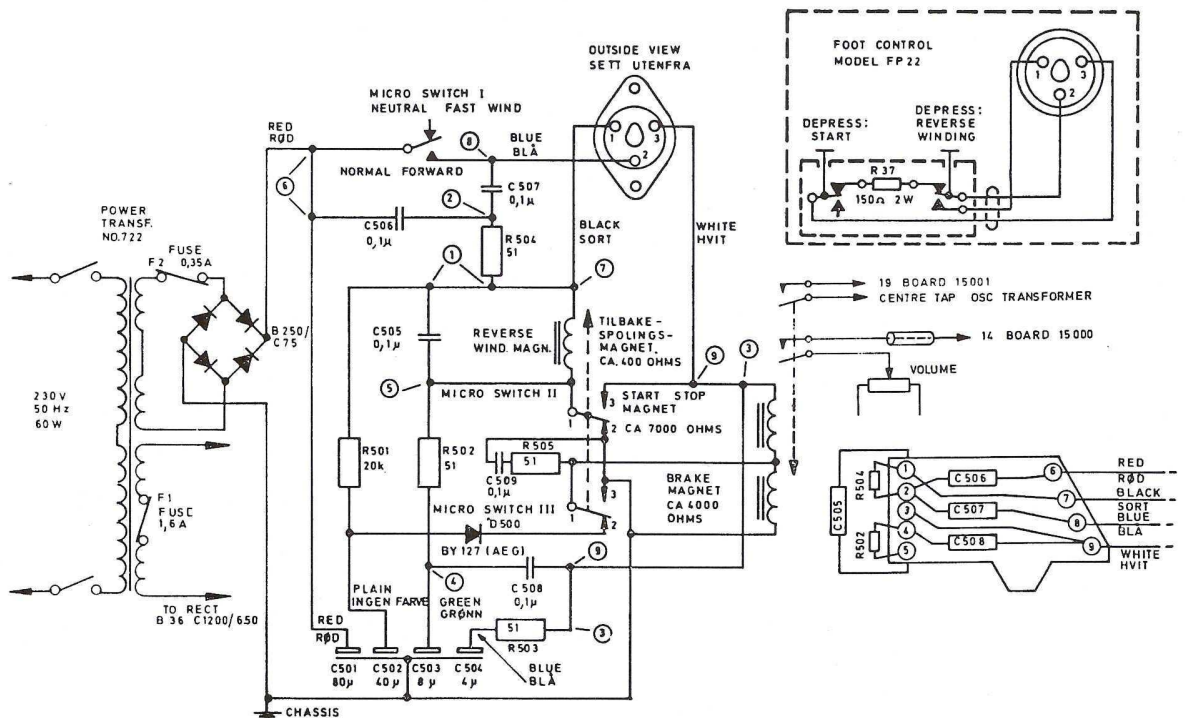
Skjema for fjernstyringsenhet modell 15 F. Over serienr. 2 510 020.
