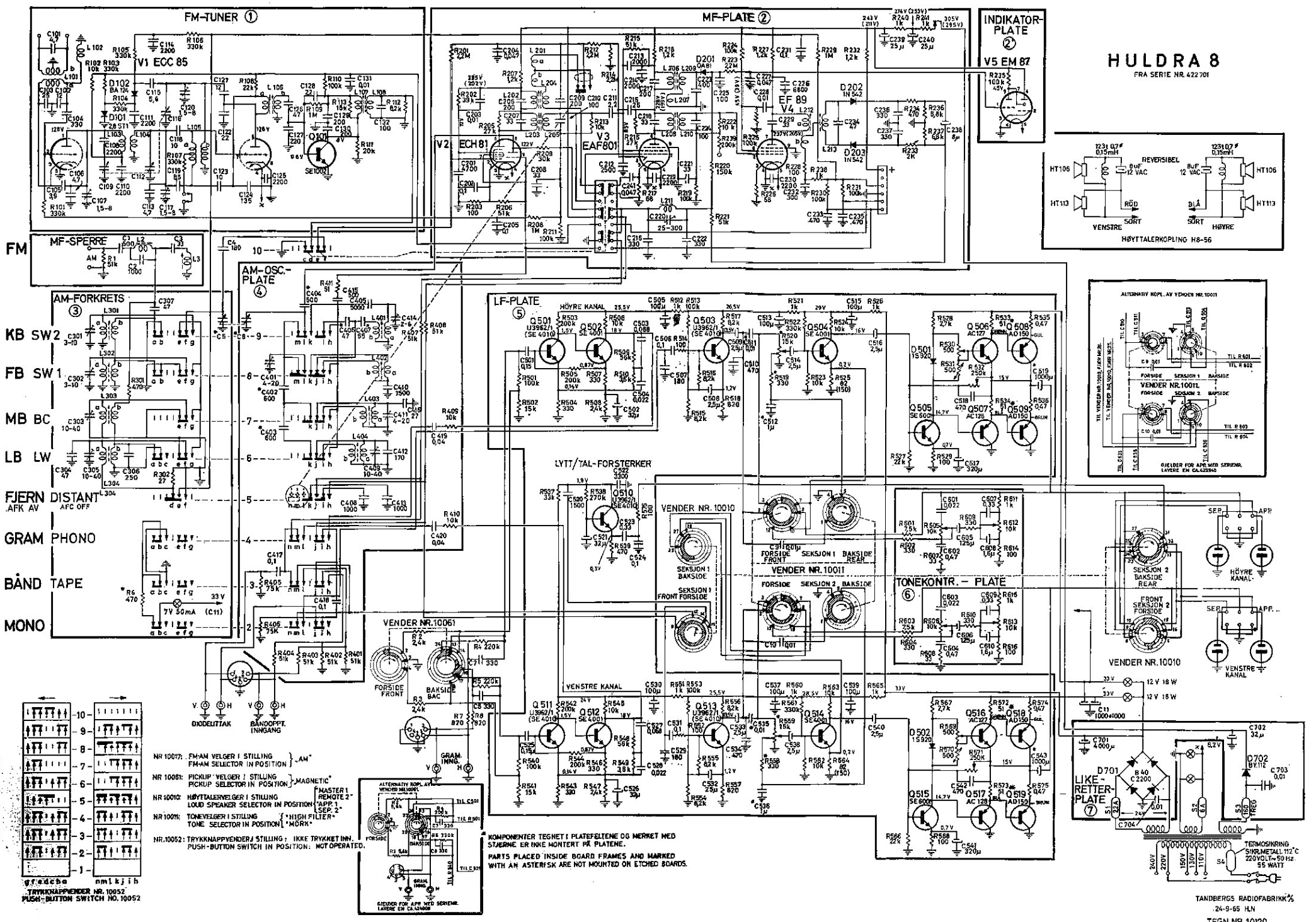
Fig. 52. Hovedskjema
