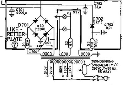
Fig. 52. Hovedskjema
