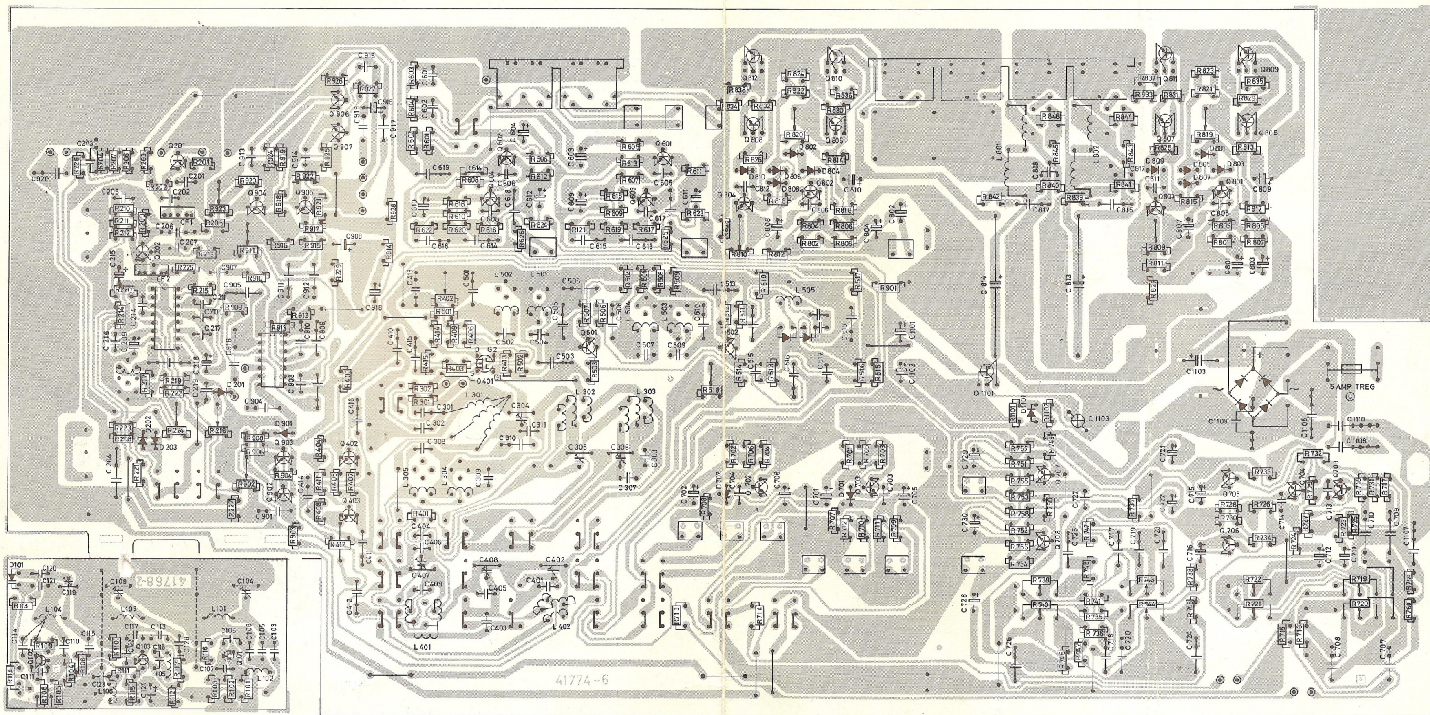
FM-tuner, sett fra foliesiden.
