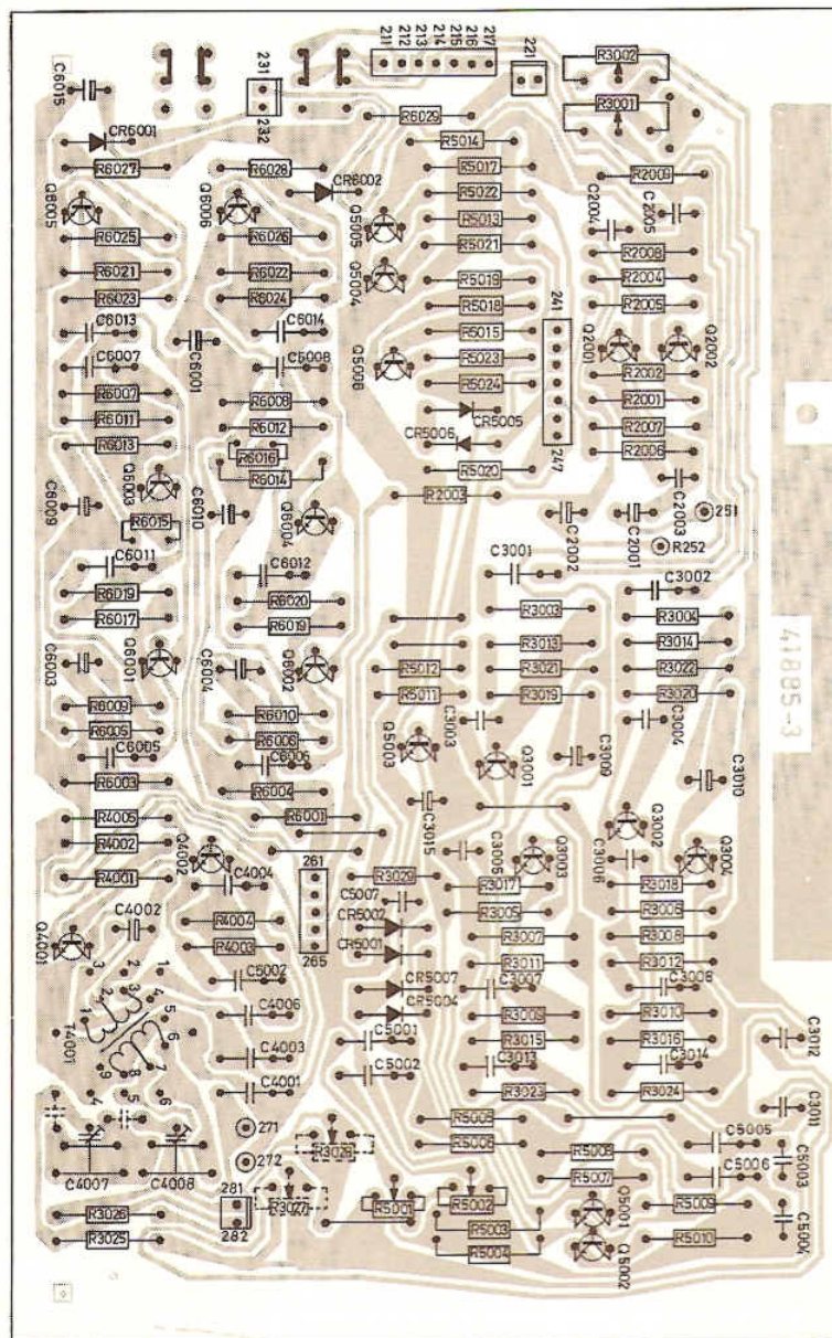
Inn/avspillingsplate, sett fra loddessiden
