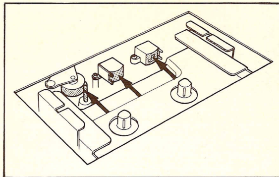
Rensing av båndløp
