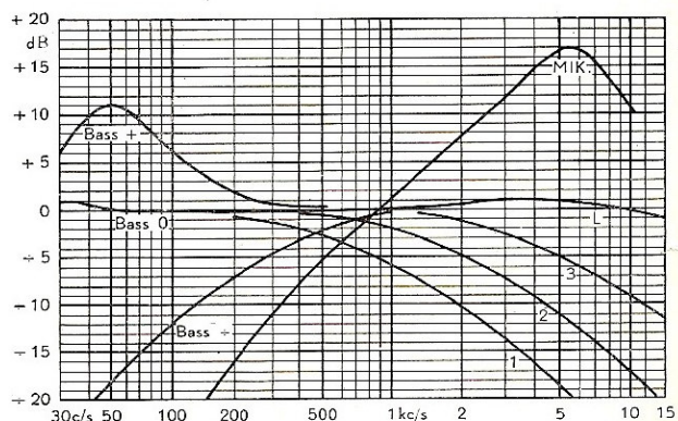
Fig. 24. Frekvenskurver for grammofon- og mikrofonforsterker. Grammofonkurver ved inng.spennings 0.25 V og uteffekt 50 mW ved 400 c/s. Mikrofonkurve ved inng.spennings 1.5 mV og uteffekt 50 mW ved 400 c/s. ÷ Bass, L-diskant og volumkontroll på maks.
