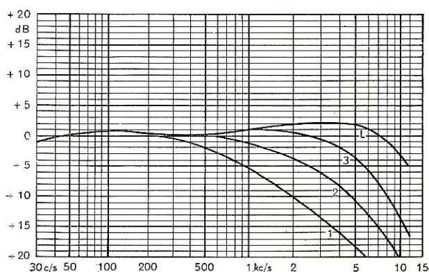
Fig. 6. Frekvenskurver for gramfonforsterker. Inng.spennning 0,25 V og uteffekt 50 mW ved 400 c/s.
