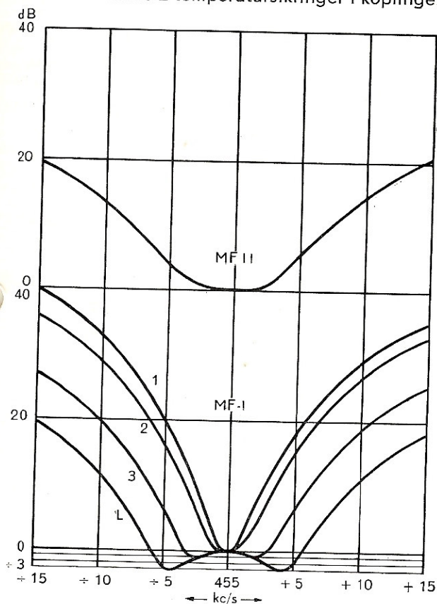
Fig. 27. Kurver for første og annet mellomfrekvensfilter for 455 kc/s. Felles kurver for Sølvsuper 6 - serien.
