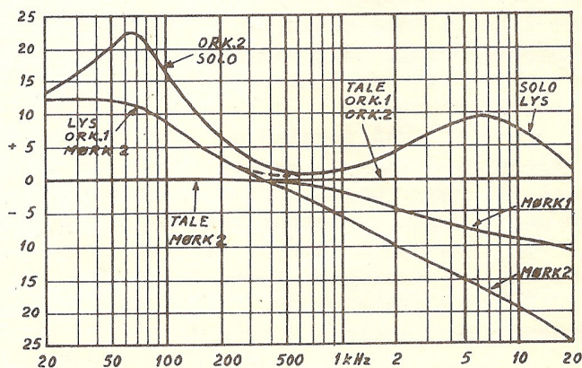
Fig. 6. Frekvenskurver for LF del målt i stilling Bånd og Gram. Signalspenning 0.25 volt. Volumkontroll -30 dB (stilling ca. 3\frac{1}{2} ). Kurvene gjelder også i stilling FM når senderen har standard preemphasis. (50 \mu s ).
