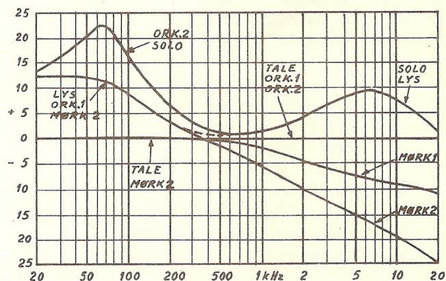
Fig. 6. Frekvenskurver for LF del målt i stilling Bånd og Gram. Signalspenning 0.25 volt. Vol. uankontroll -30 dB (stilling ca. 3 1/2). Kurvene gjelder også i stilling FM når senderen har standard preemphasis. (50 µs).
