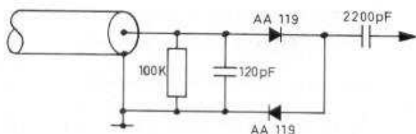
Fig. 9. Diodeprobe.
