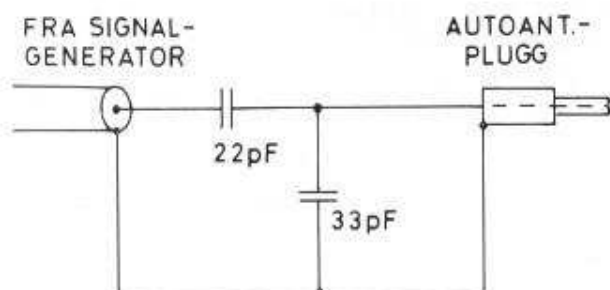
Fig. 6. Ekvivalent bilantenne.
