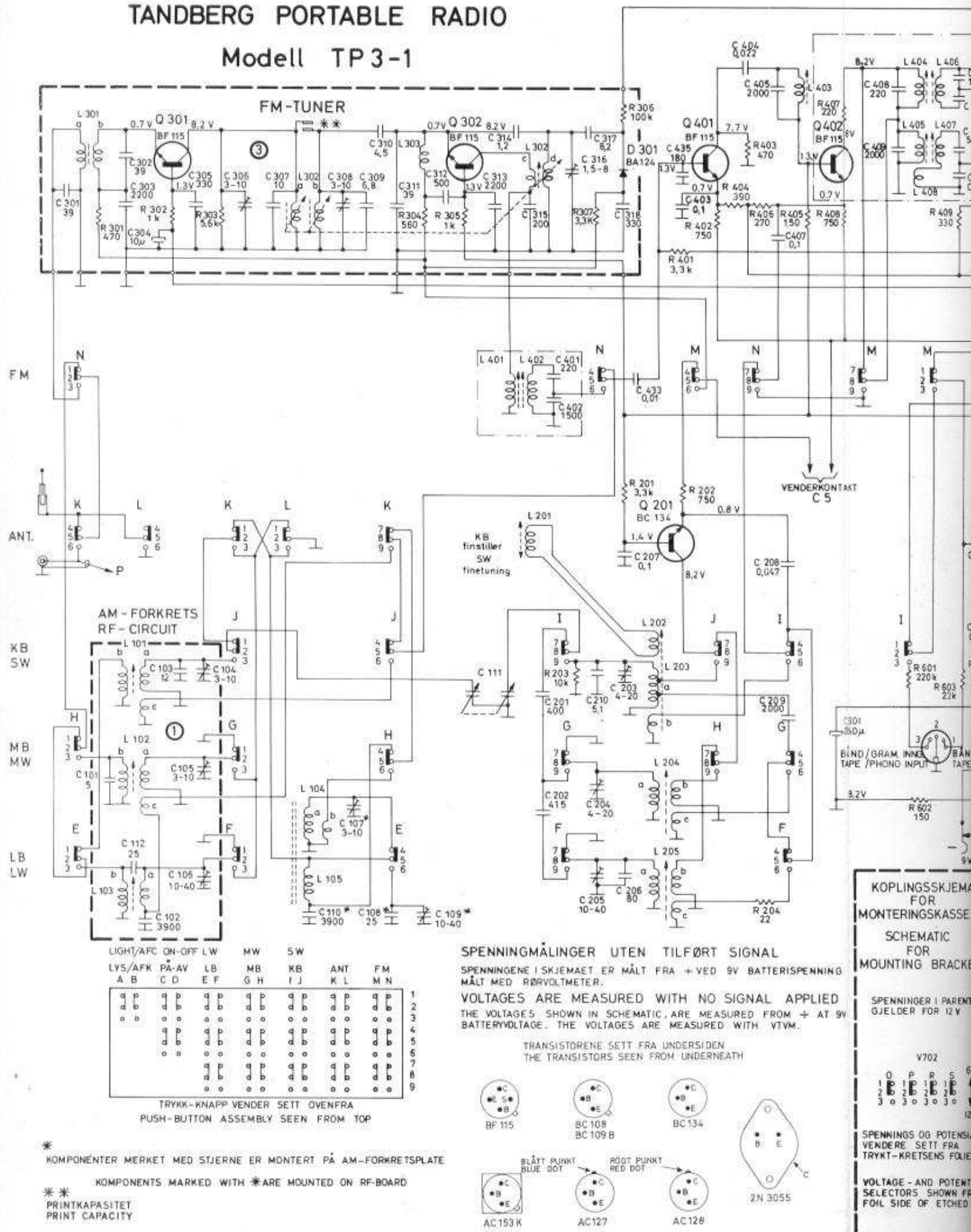
Fig. 22. Hovedskjema TP3-1.
