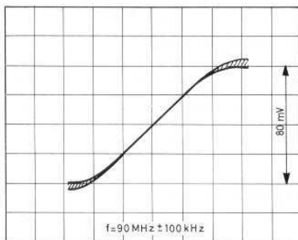
Fig. 13. Diskriminatorkurve.
