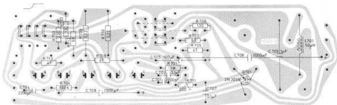
Fig. 26. Plate for monteringskassett sett fra foliesiden.
