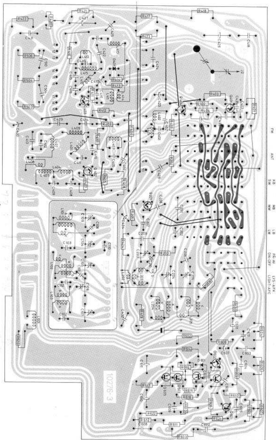
Fig. 21. Hovedplaten og forkretsplaten sett fra foliesiden. Venderplaten er trykt i rødt.
