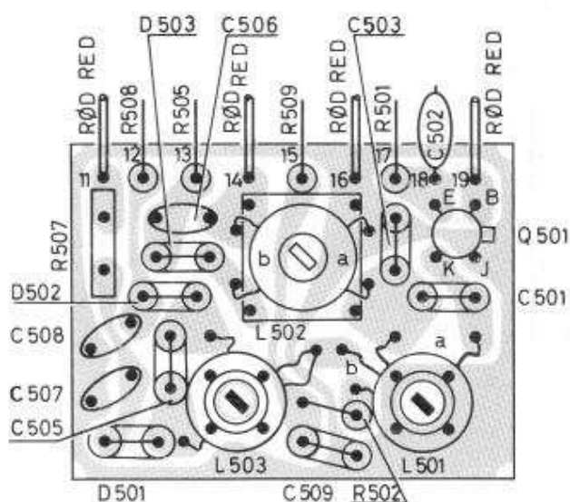
Fig. 25. Detektorplaten sett fra komponentsiden.
