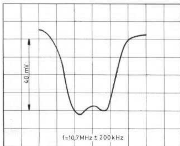
Fig. 10. FM—MF-kurve.
