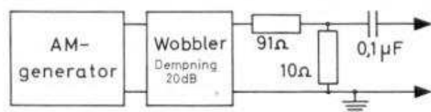
Fig. 4. Måleoppstilling for AM-trimming.
