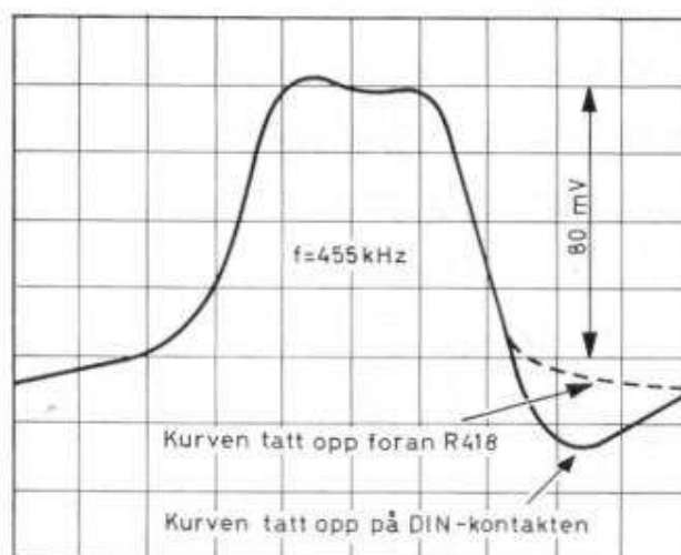
Fig. 5. AM—MF-kurve.
