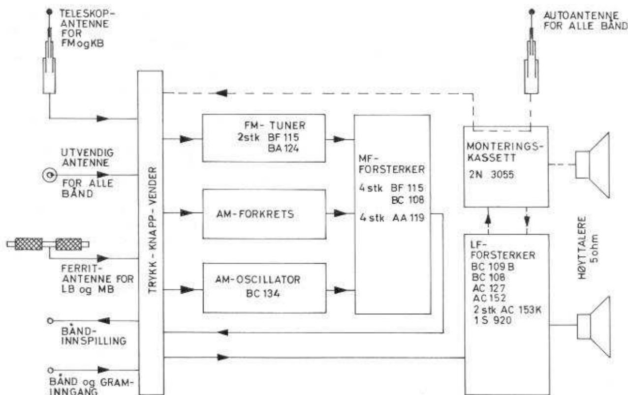
Fig. 1. Blokkskjema TP3-1.
