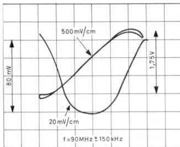
Fig. 12. FM—MF + diskriminator.
