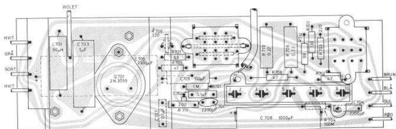
Fig. 27. Plate for monteringskasset sett fra follesiden.
