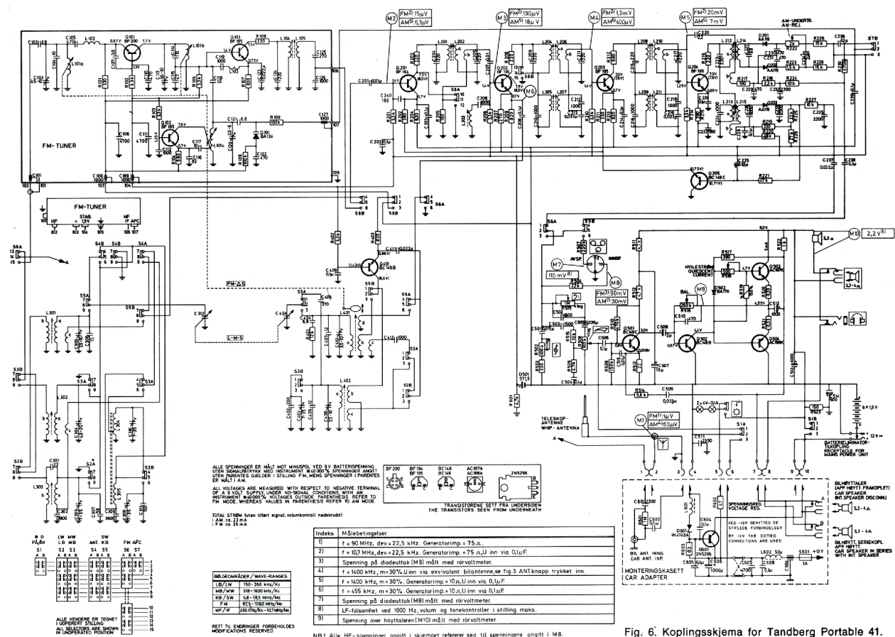
Fig. 6. Kopleingsskjema for Tandberg Portable 41.
