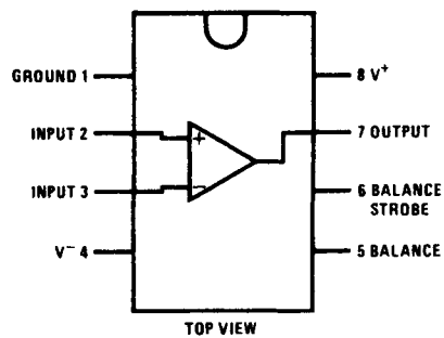
U901 MLM311
