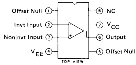
U401 MC1741CP
