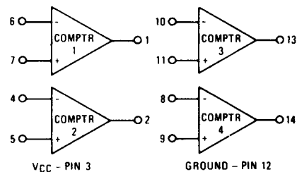
U702 MC3302
