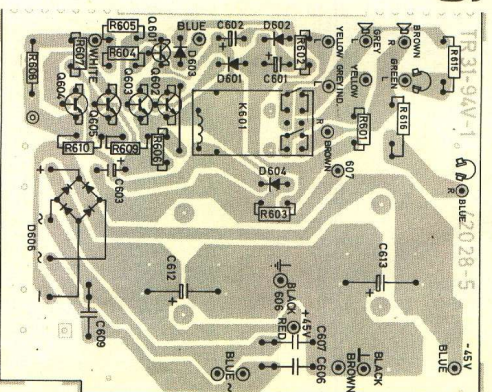
Sett fra foliesiden
