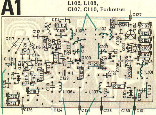
C118, FM-osc. L106, L107, FM-MF L101, C103, Forkrets Sett fra foliesiden
