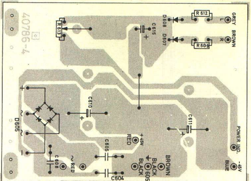
Sett fra foliesiden
