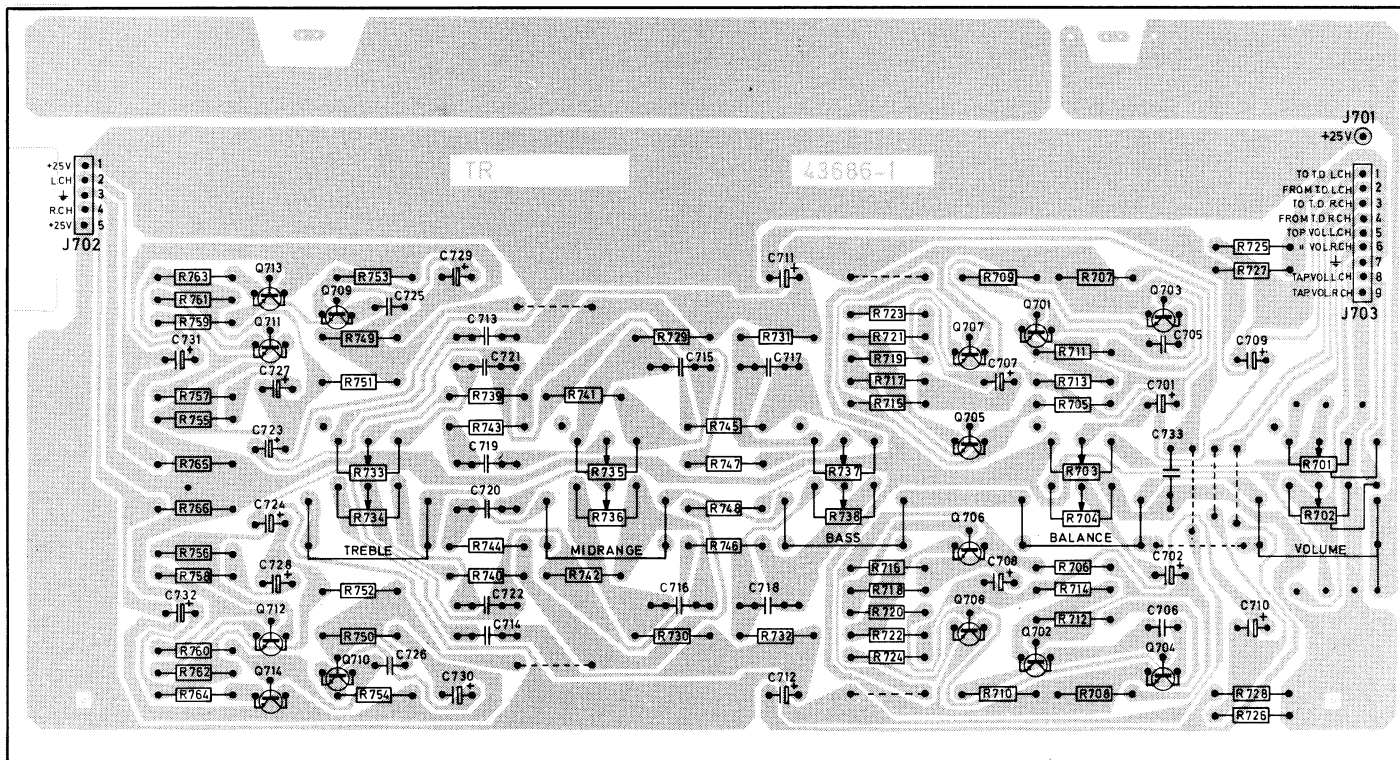
PW-BRD, PREAMPLIFIER/TONE CONTROL TL-KORT, FORFORSTERKER/TONEKONTROLL
