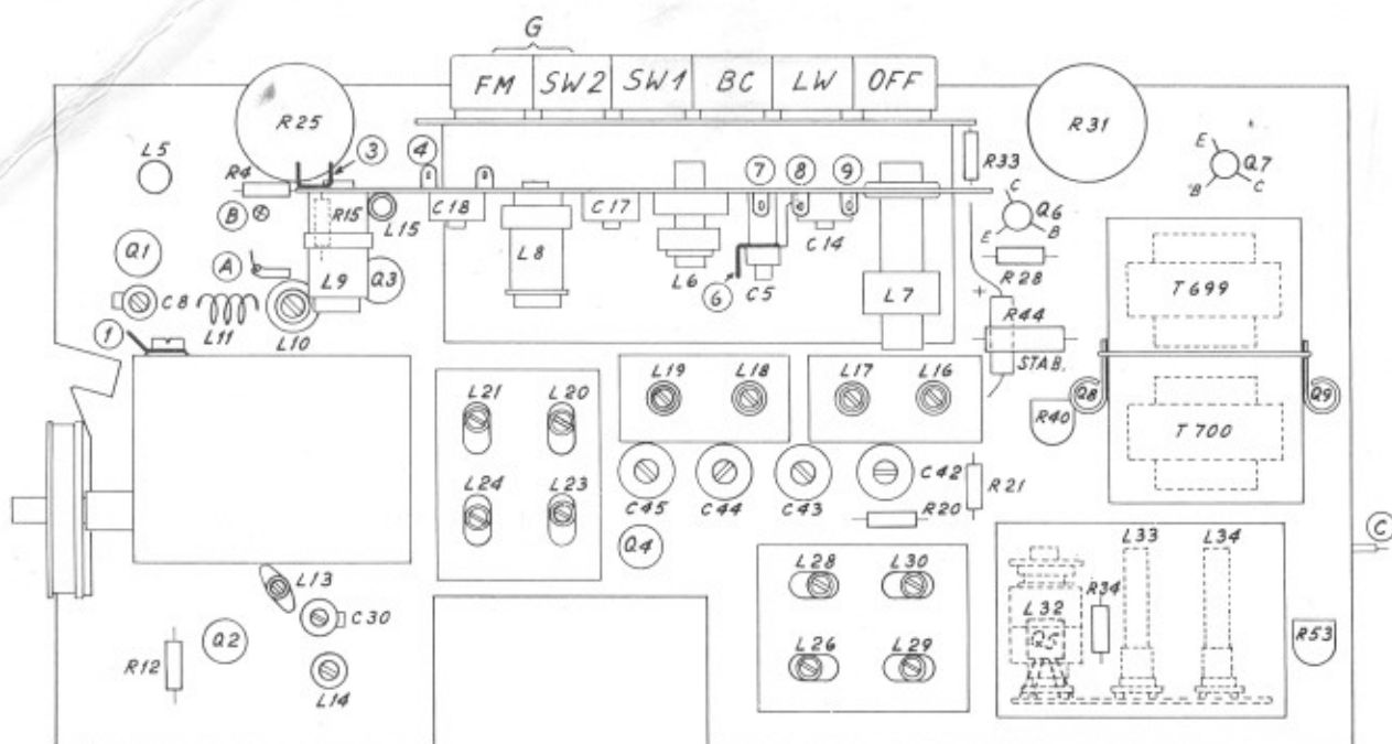
Fig. 6. TTR 1 layout.
