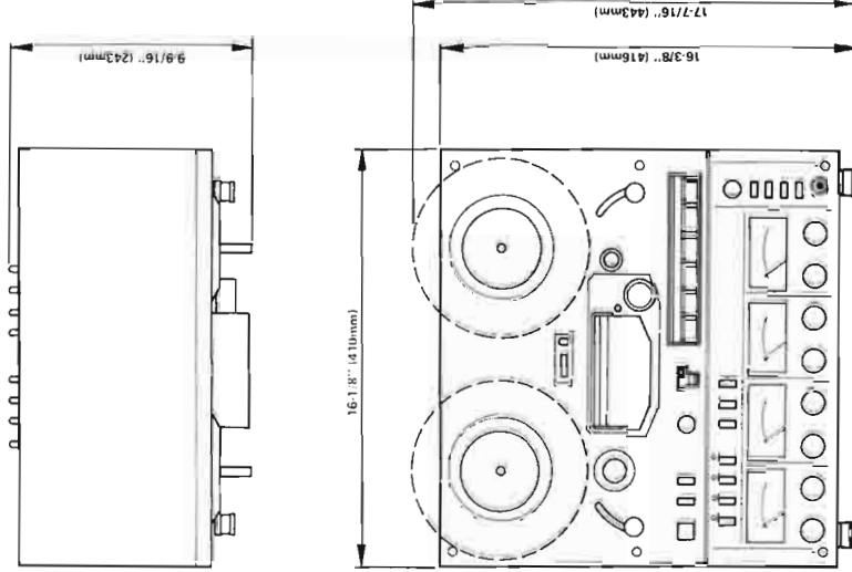
Fig. 2-1 Dimensions
