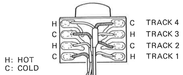
Fig. 5-5 REC/PLAY head wiring diagram 録/再ヘッド接続図
