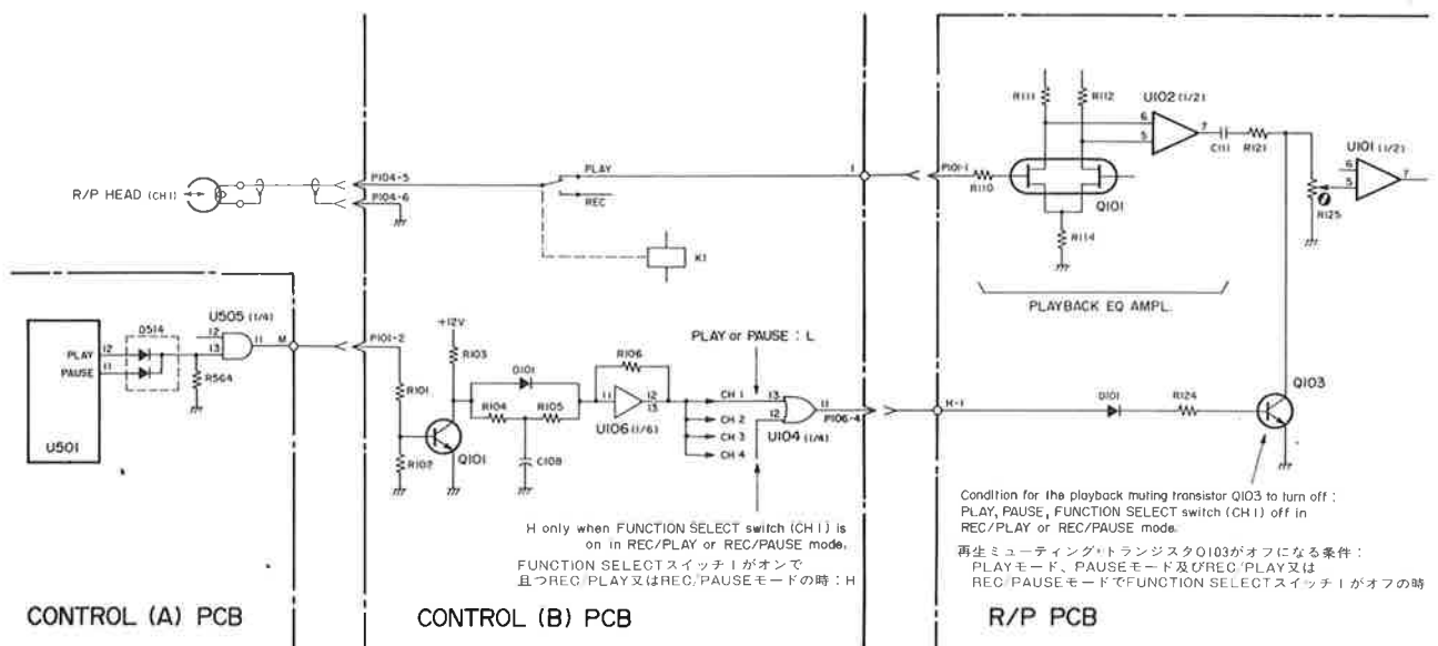
Fig. 6-14 Playback muting circuit 再生ミュート回路
