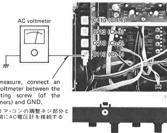
Fig. 5-7 Oscillator output check 発振器出力のチェック
