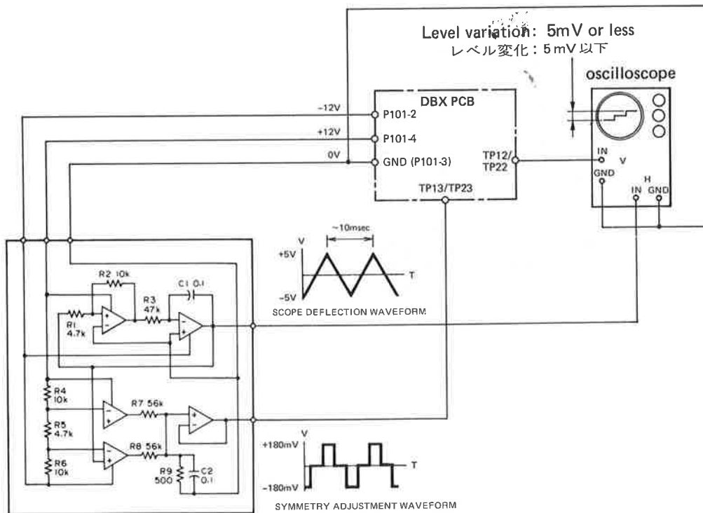
VCA symmetry adjustment waveform generator VCAシンメトリ調整用波形発振器
