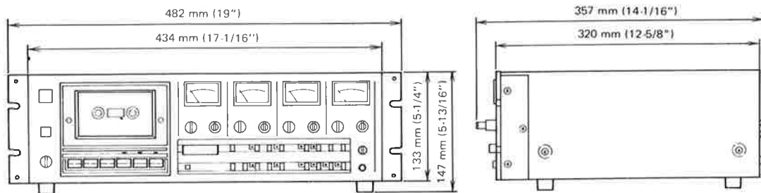
Fig. 2-2 Dimensions 寸法図
