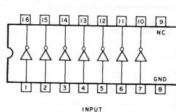
M54517P
