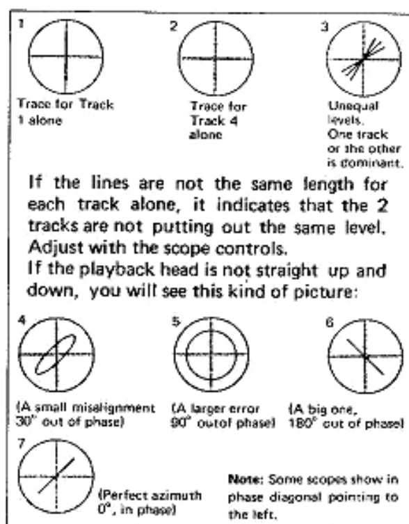
Fig. 2-11 Phase Shift
