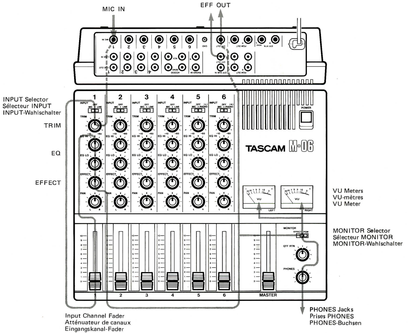
Fig. 2 EFFECT MIX SYSTEM (AND MONITOR SYSTEM) Fig. 2 SYSTEME DE MIXAGE EFFET (ET CELUI DE MONITOR) Abb. 2 EFFEKTMISCHSYSTEM (UND MONITORSYSTEM)
