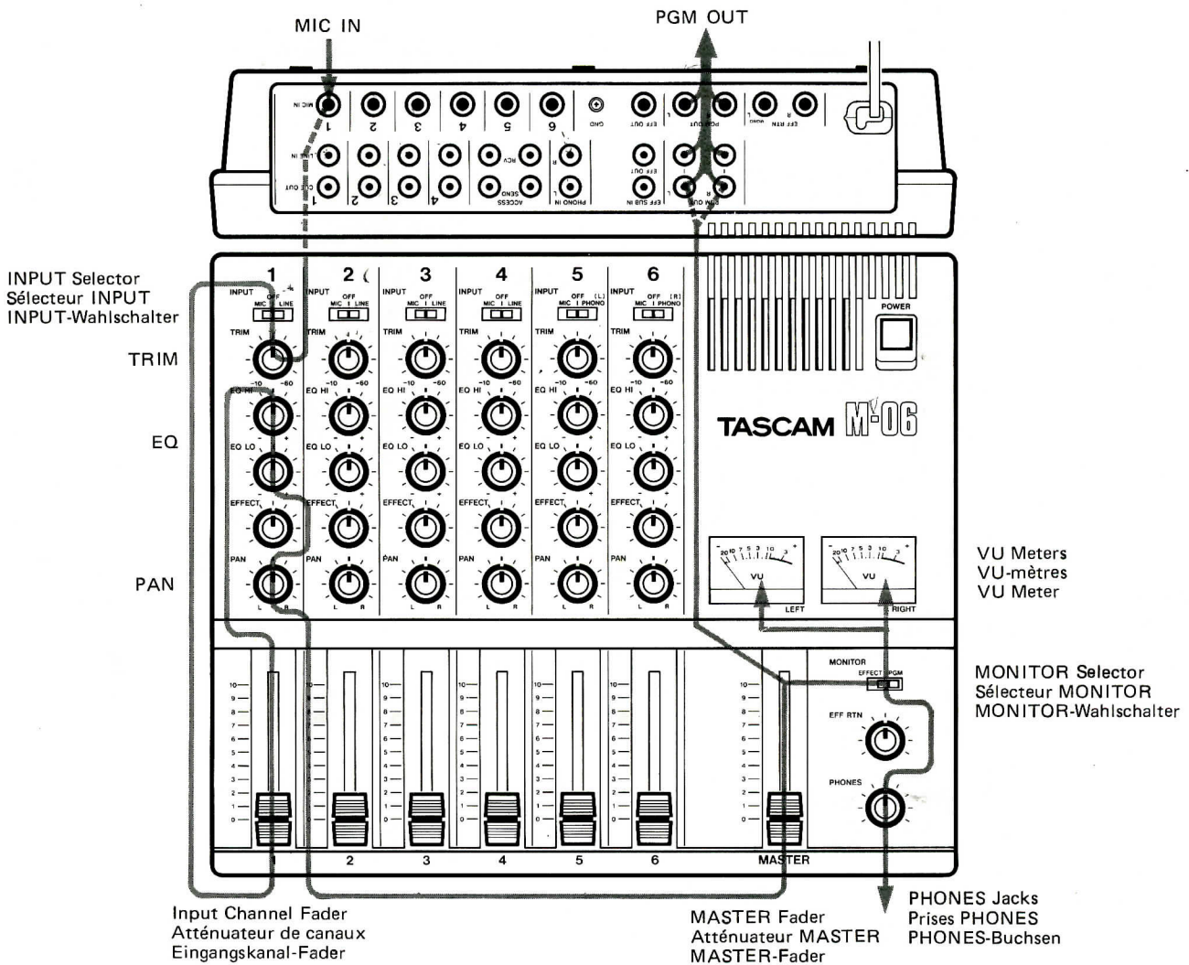
Abb. 1 HAUPTMISCHSYSTEM (UND MONITORSYSTEM)
