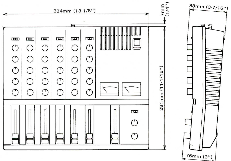
Fig. 12 EXTERNAL DIMENSIONS Fig. 12 DIMENSIONS EXTERIEURES Abb. 12 ABMESSUNGEN
