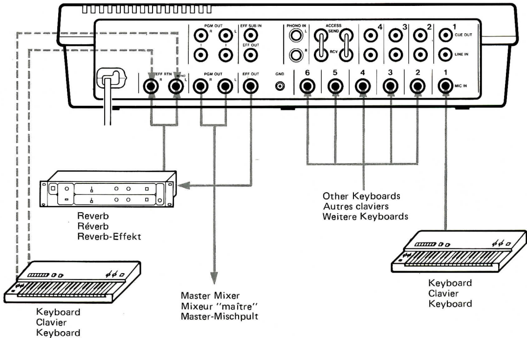
Fig. 9 USING AS A KEYBOARD SUB-MIXER AND SYSTEM EXPANSION Fig. 9 UTILISATION EN TANT QUE SOUS-MIXEUR POUR CLAVIERS ET EXPANSION DE SYSTEME Abb. 9 VERWENDUNG ALS KEYBOARD-SUBMIXER UND SYSTEMERWEITERUNG
