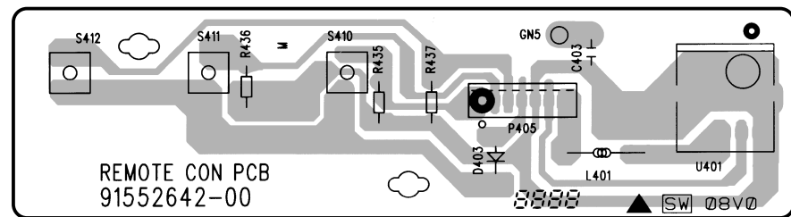
REMOTE CON PCB
