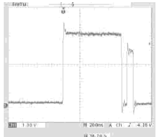
2. ROM- DATA-BUS
