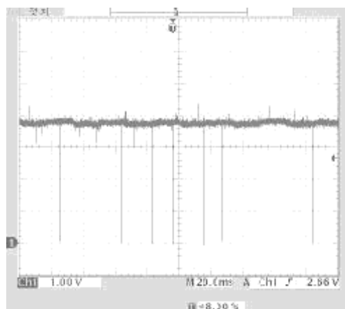
19. VFD-CLK
