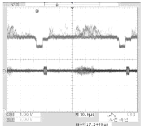
23. S-VIDEO
