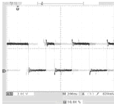
22. OPTICAL-OUT
