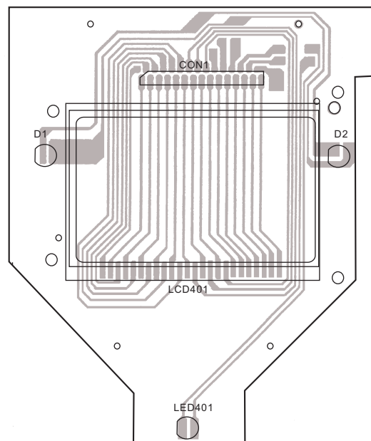
DISPLAY PCB
