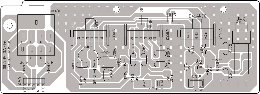
EQ PCB
