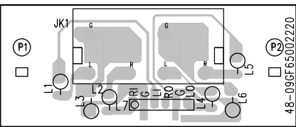
AUX PCB
