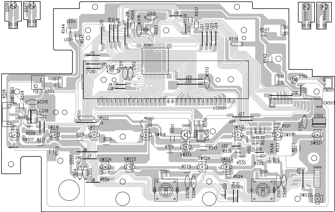
DISPLAY PCB
