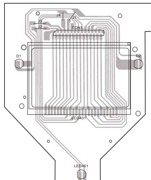
DISPLAY PCB
