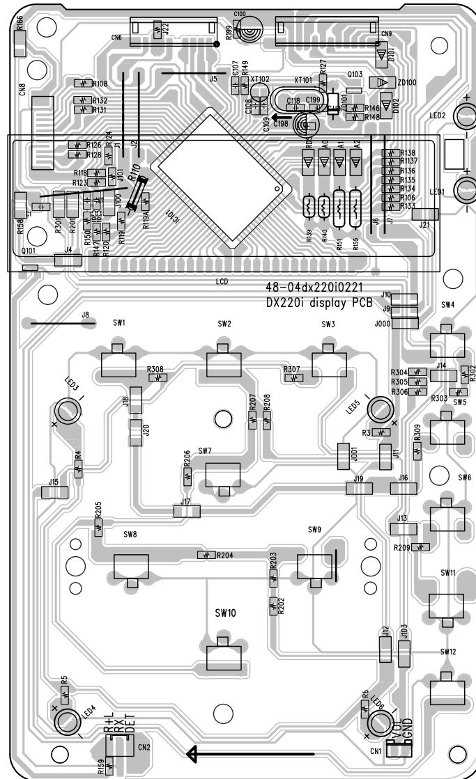
DISPLAY PCB
