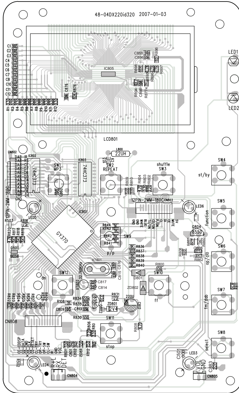
DISPLAY PCB
