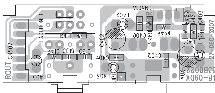
AUX PCB
