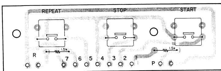
FUNCTION SW PCB (P-9)
