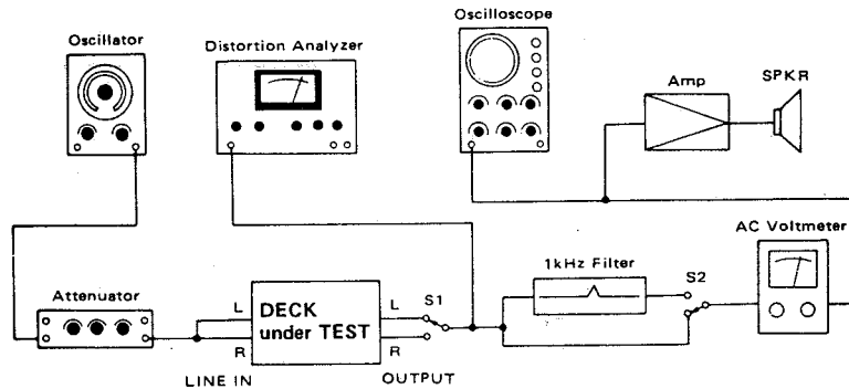
Fig. 5-2 Basic test setup 基本測定接続図
