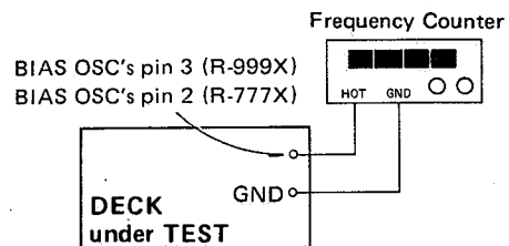
Fig. 5-8 Test setup for bias osc. frequency adjustment バイアス発振周波数調整用接続図
