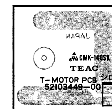
T-MOTOR PCB
