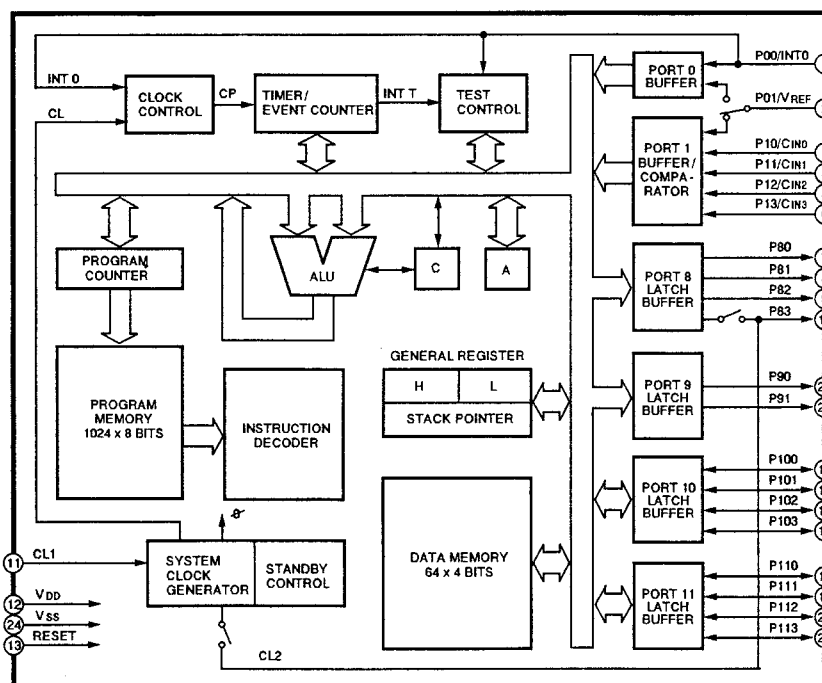
U501 uPD7566CS
