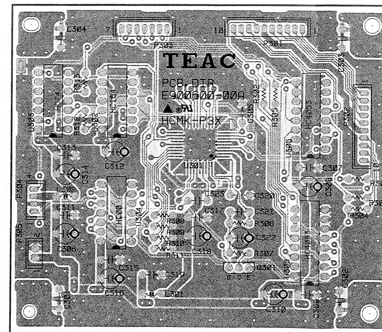
DIR PCB
