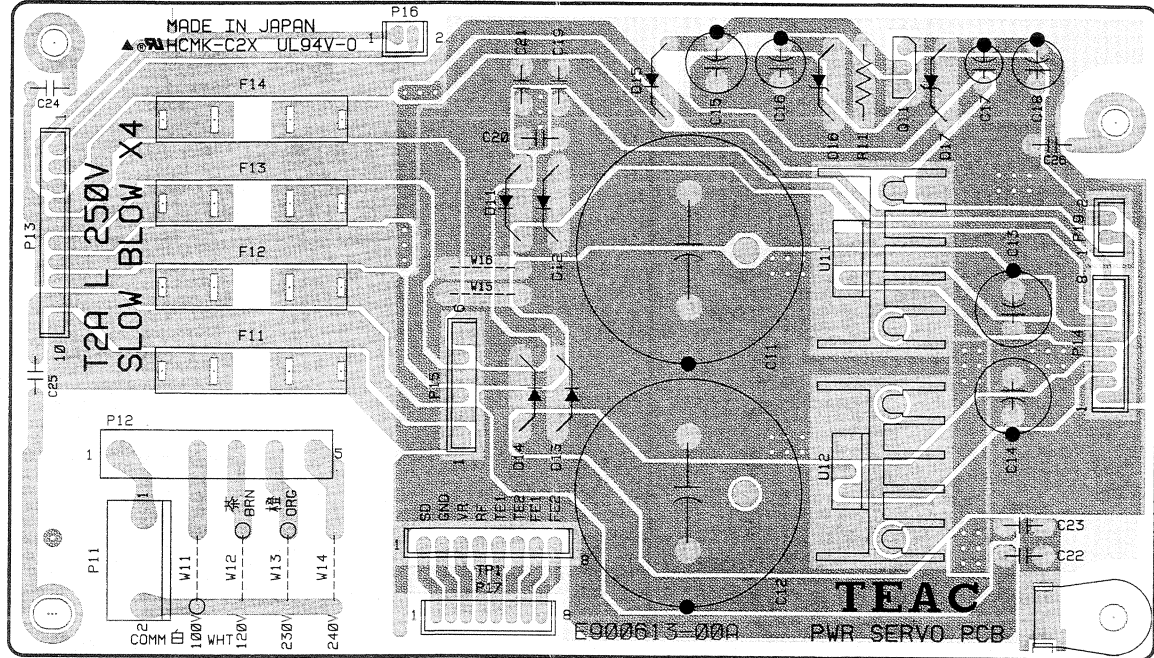
PWR-SERVO PCB
