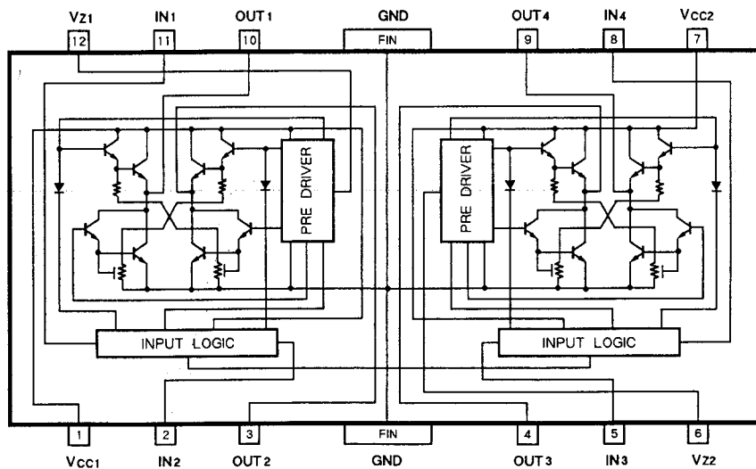
U410 LB1649
