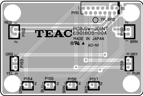
SW-JOINT PCB
