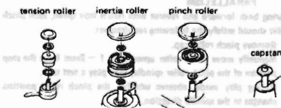
Fig. 2-27
