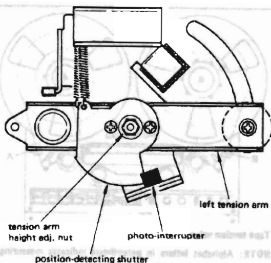
Fig. 2-11
