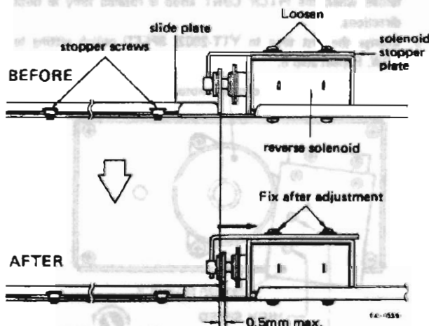
Fig. 2-26
