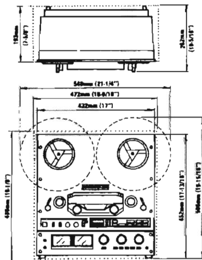
Fig. 1-1 Dimensions
