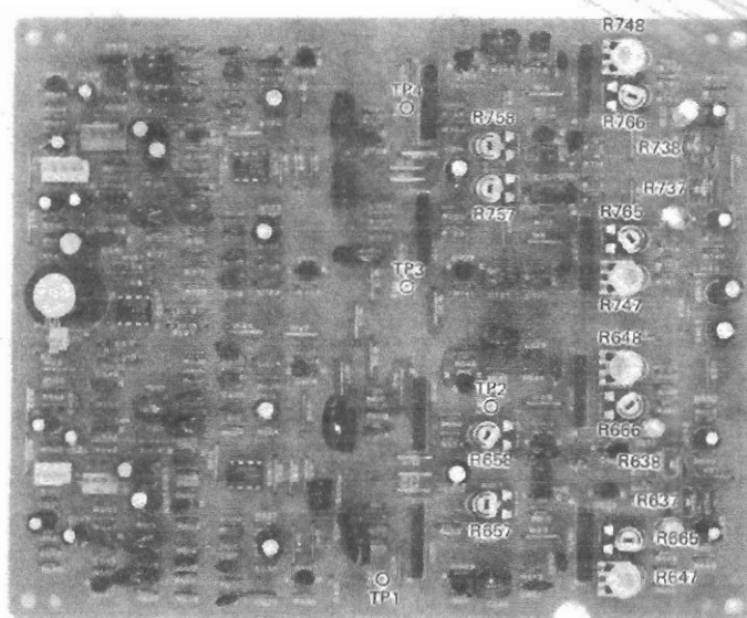
Fig. 3-14 DBX PCB
