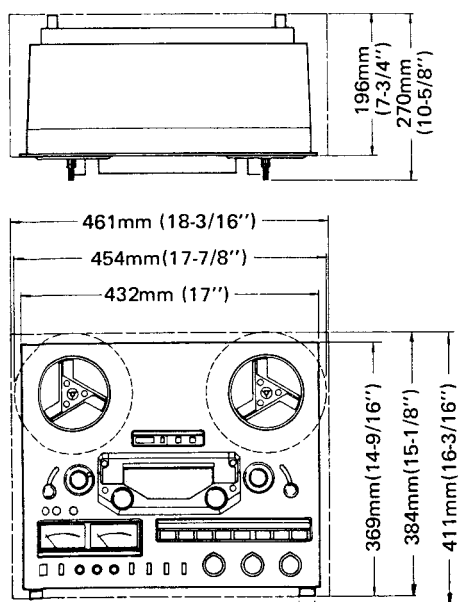
Fig. 1-1 Dimensions
