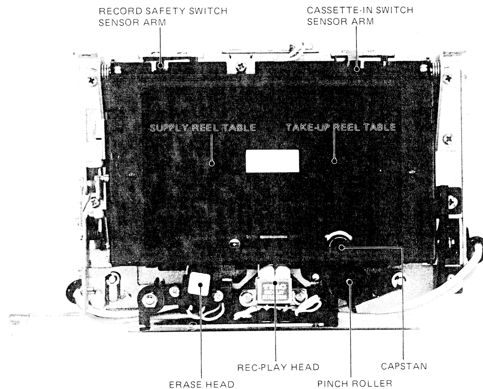
Fig. 3-2 Transport view (トランスポート)
