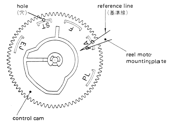
Fig. 5-6 Control cam positioning (コントロール・カムの位置調整)
