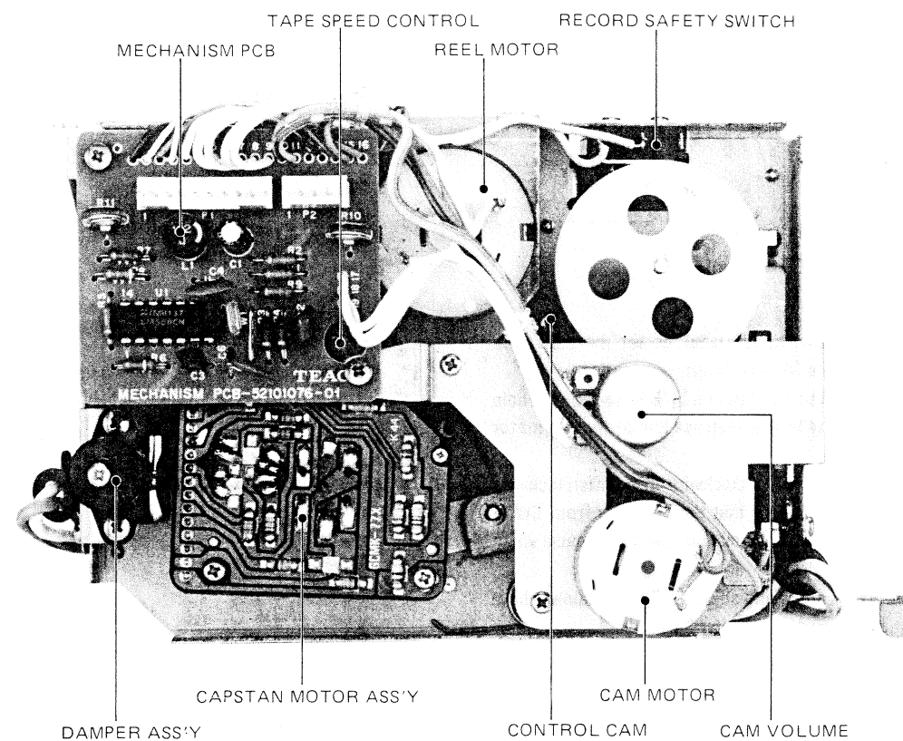
Fig. 3-3 Transport rear view (トランスポート裏面)
