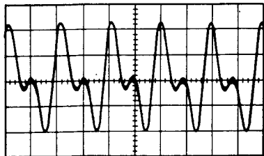
Fig. 6-15 RMS SYM check (Incorrect) (RMS SYM 不良)
