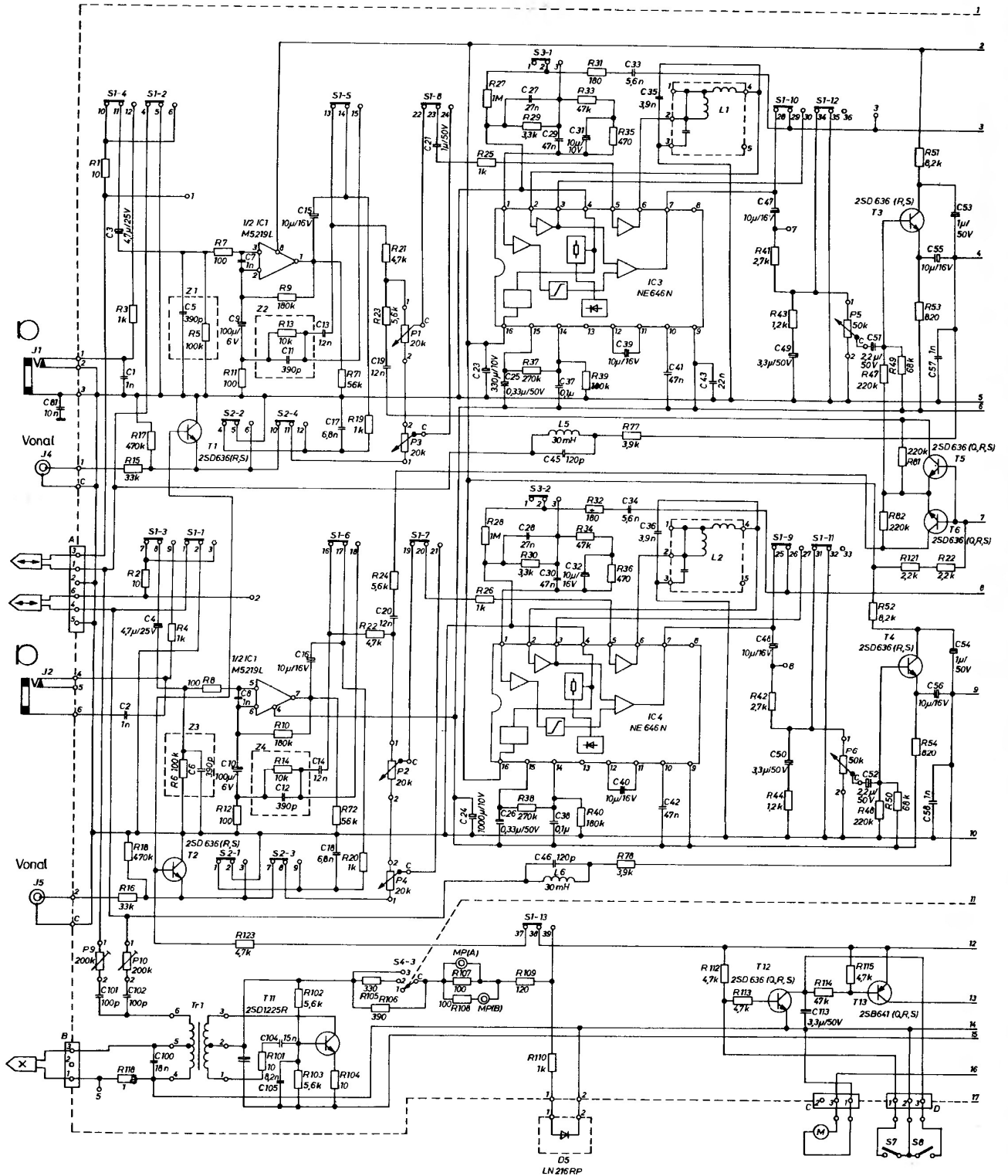
176. ábra A Technics M 216 áramköreinek kapcsolási vázlata
