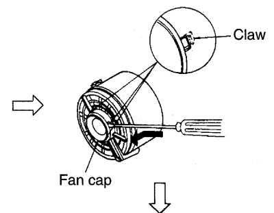
Step 3 Remove the fan cap.
