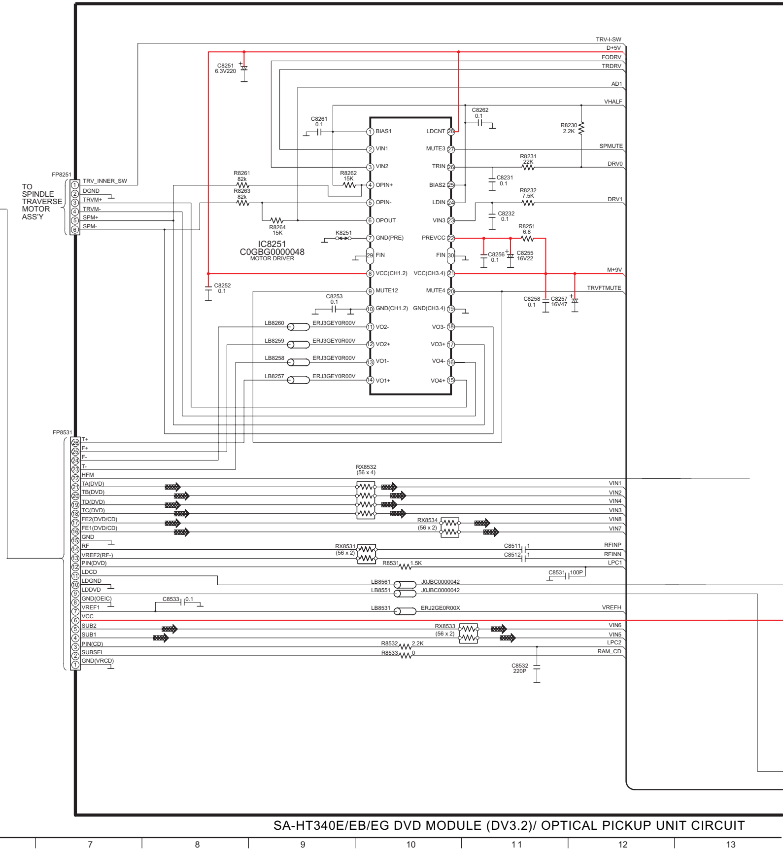
A DVD MODULE (DV3.2) CIRCUIT : +B SIGNAL LINE : CD-DA SIGNAL LINE
