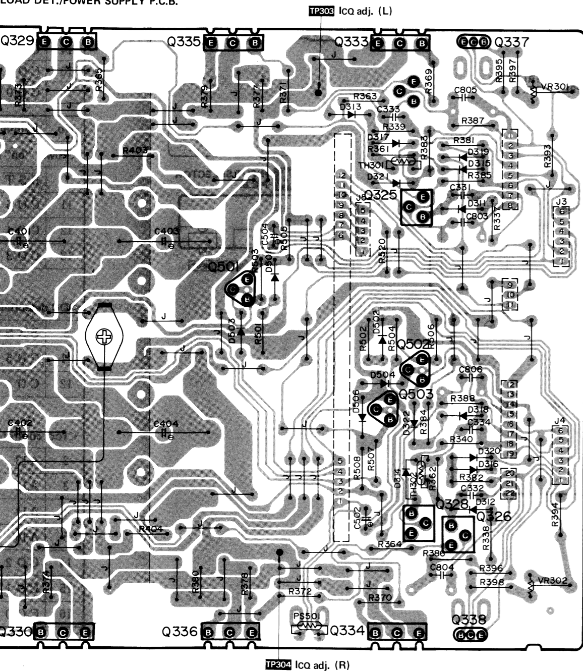
LOAD DET./POWER SUPPLY P.C.B.
