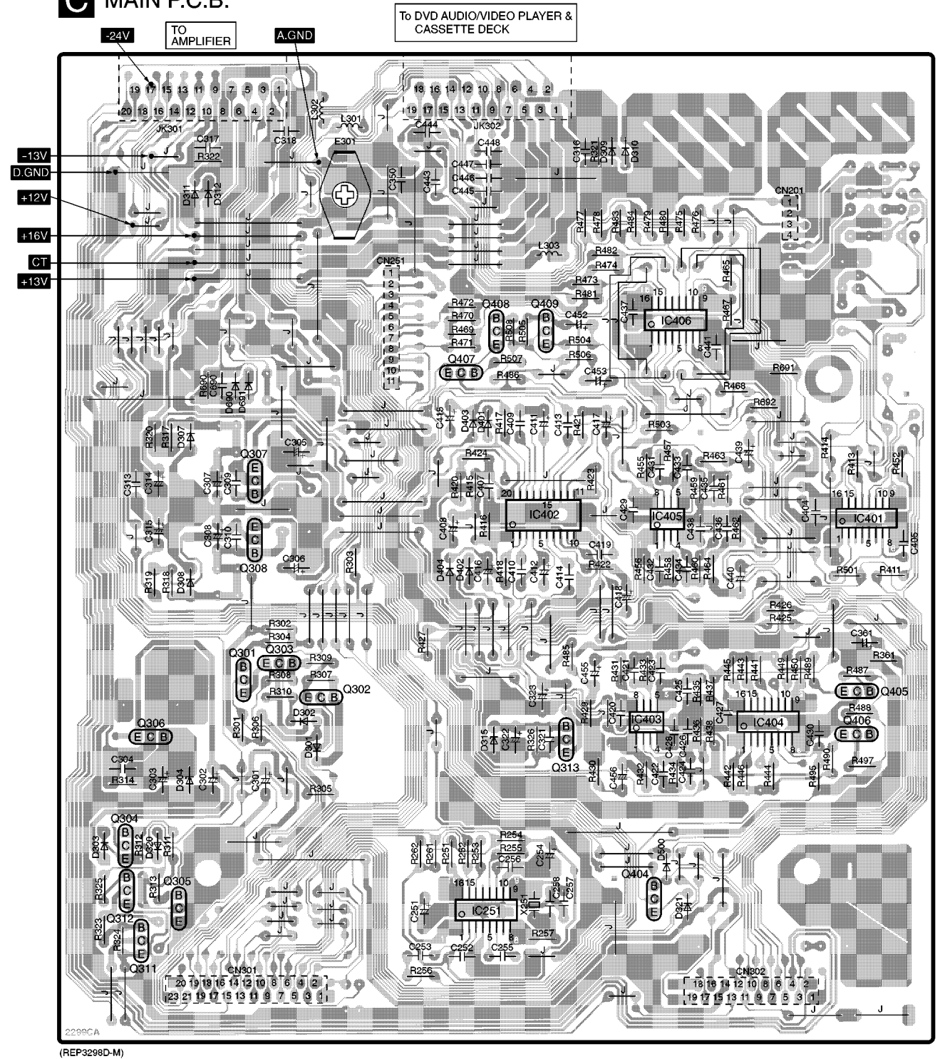
C MAIN P.C.B.
