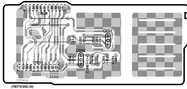
D CONNECTOR P.C.B.
